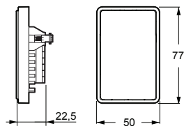
IHC CONTROL® Alarm Sløjfeindsats LK FUGA
