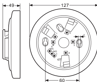
IHC CONTROL® Alarm Røgsensor optisk
