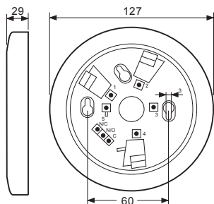
IHC CONTROL® Alarm Røgsensor Relæsokke til røg-sensor
