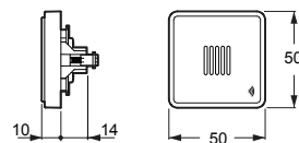
IHC CONTROL® indsats lyd giver 24 V DC 80DB med sikring LK FUGA
