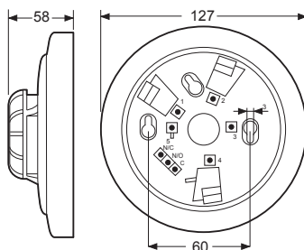
IHC CONTROL® Alarm Røgsensor optisk / termisk
