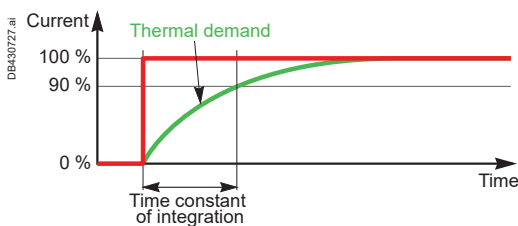
Thermal demand
