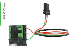
ESM: ERMS switch module
